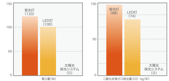
太陽光採光システムの省エネルギー効果
