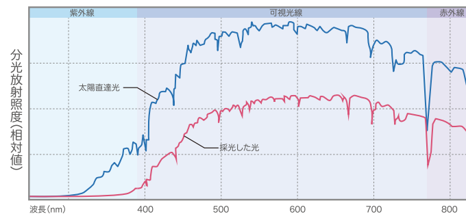
太陽直達光と採光した光
