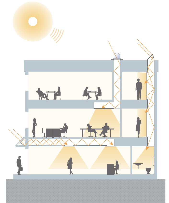
光ダクト方式
