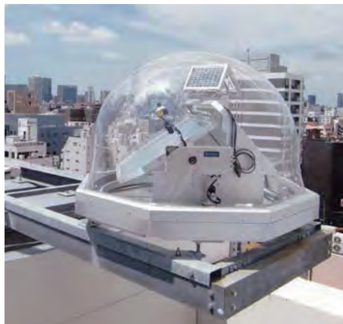
プリズム・ミラー併用方式、ミラー方式
