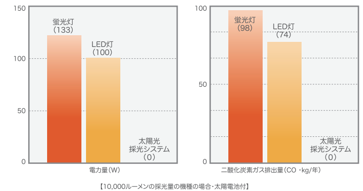
太陽光採光システムの省エネルギー効果
